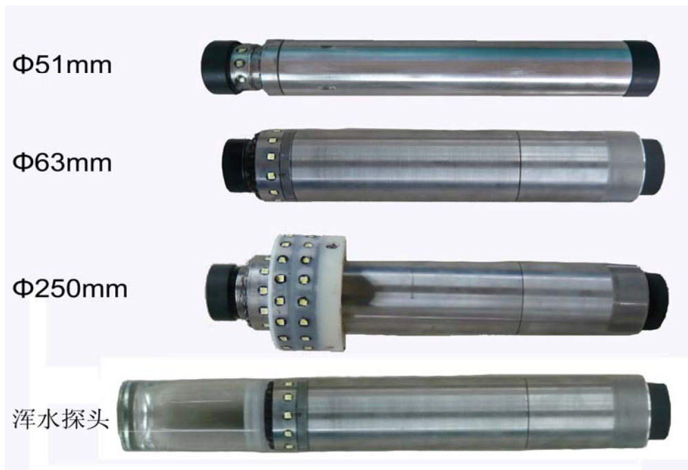
图 8 探头外观
