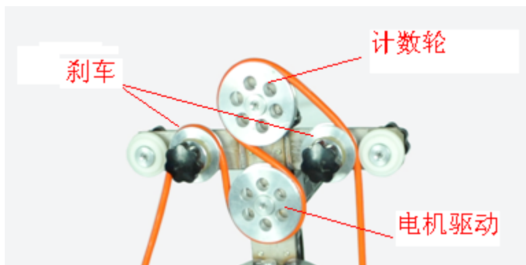
图6 电机与轮毂（图右侧连下井探头）
